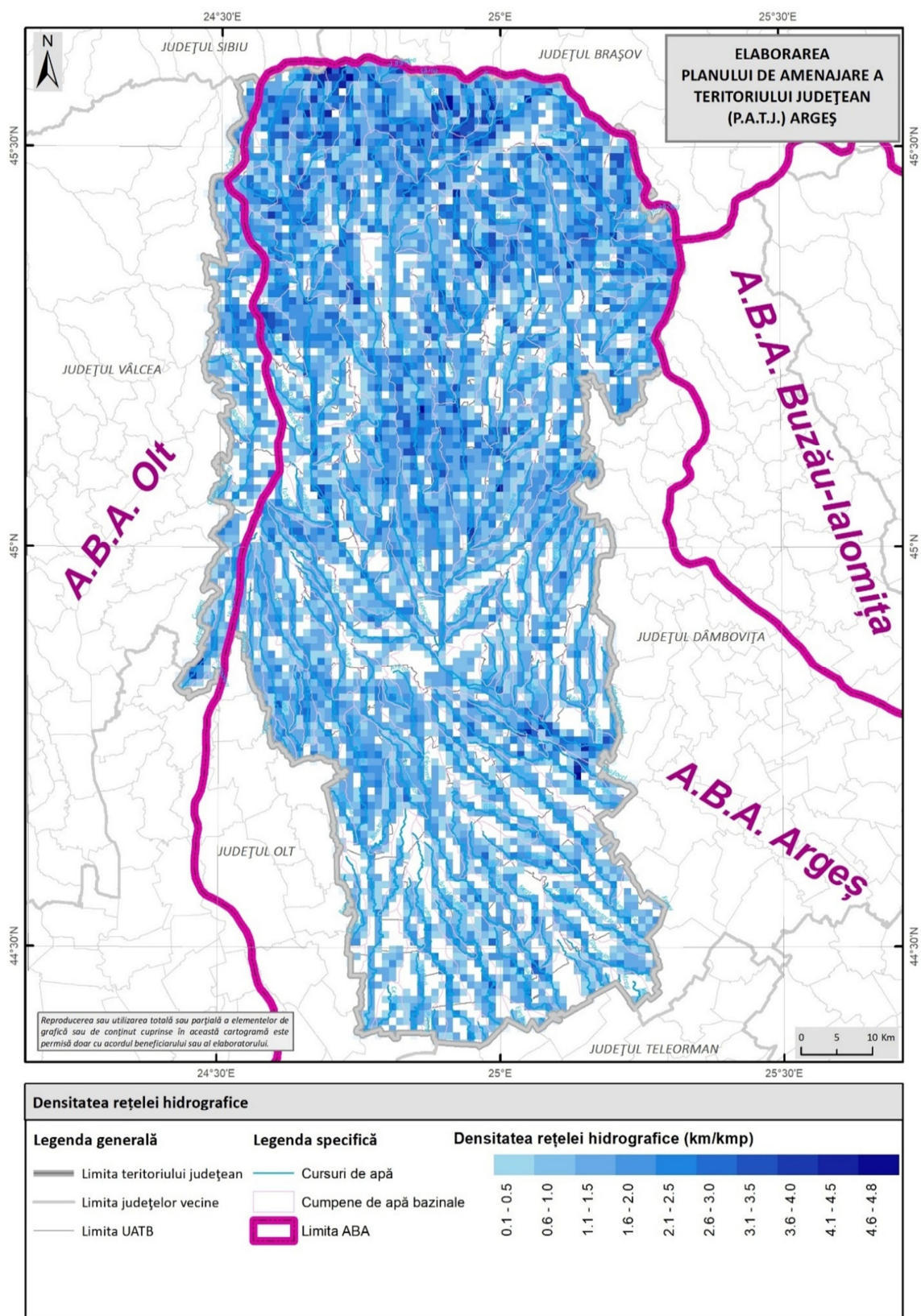
DENSITATEA REȚELEI HIDROGRAFICE DIN JUDEȚUL ARGEȘ
