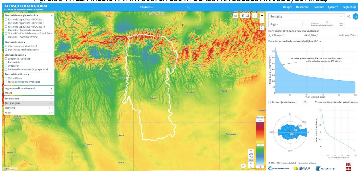
Fig. 2.93 VITEZA MEDIE A VÂNTULUI LA 100 M DEASUPRA SOLULUI ÎN JUDEȚUL ARGEȘ
