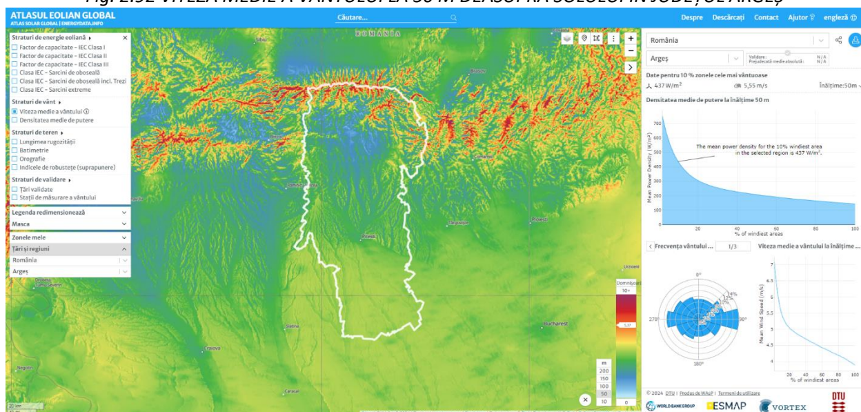
Fig. 2.92 VITEZA MEDIE A VÂNTULUI LA 50 M DEASUPRA SOLULUI ÎN JUDEȚUL ARGEȘ
