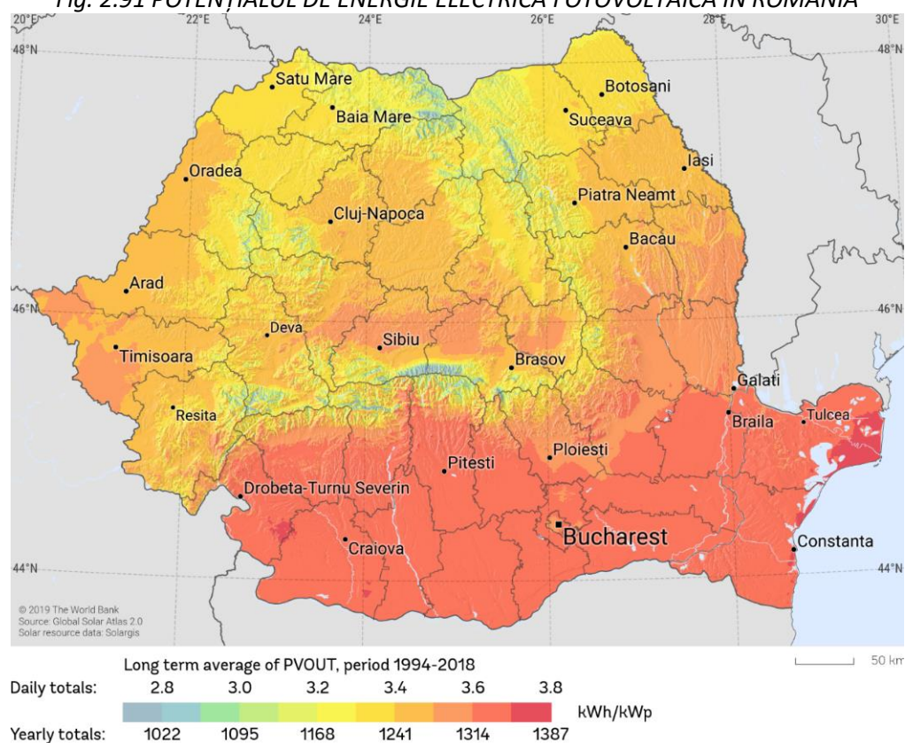
Fig. 2.91 POTENȚIALUL DE ENERGIE ELECTRICĂ FOTOVOLTAICĂ ÎN ROMÂNIA
