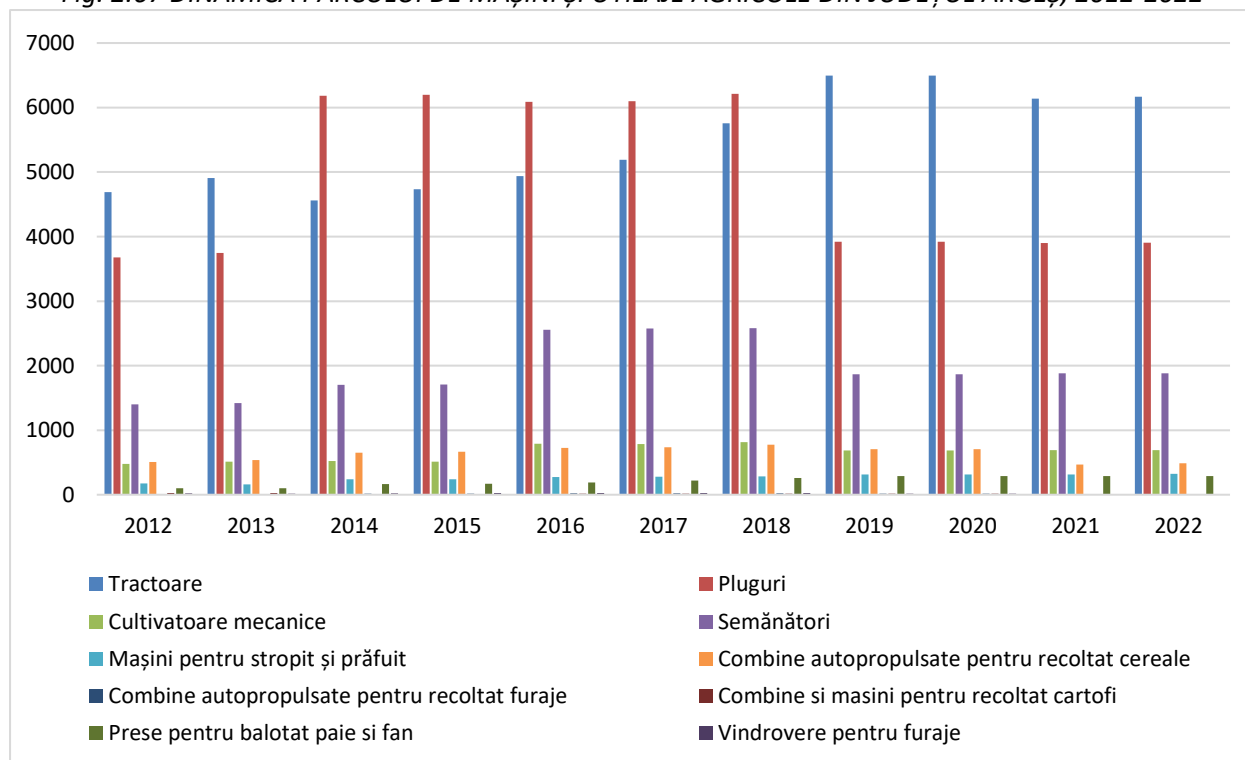
Fig. 2.67 DINAMICA PARCULUI DE MAȘINI ȘI UTILAJE AGRICOLE DIN JUDEȚUL ARGEȘ, 2012-2022
