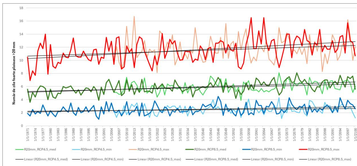
Fig. 2.23. EVOLUȚIA NUMĂRULUI DE ZILE CU PRECIPITAȚII PESTE 20 MM (FOARTE ABUNDENTE) ÎN SCENARIU RCP4,5 ȘI 8,5 ÎN JUDEȚUL ARGEȘ PENTRU PERIOADA 1971-2100.
