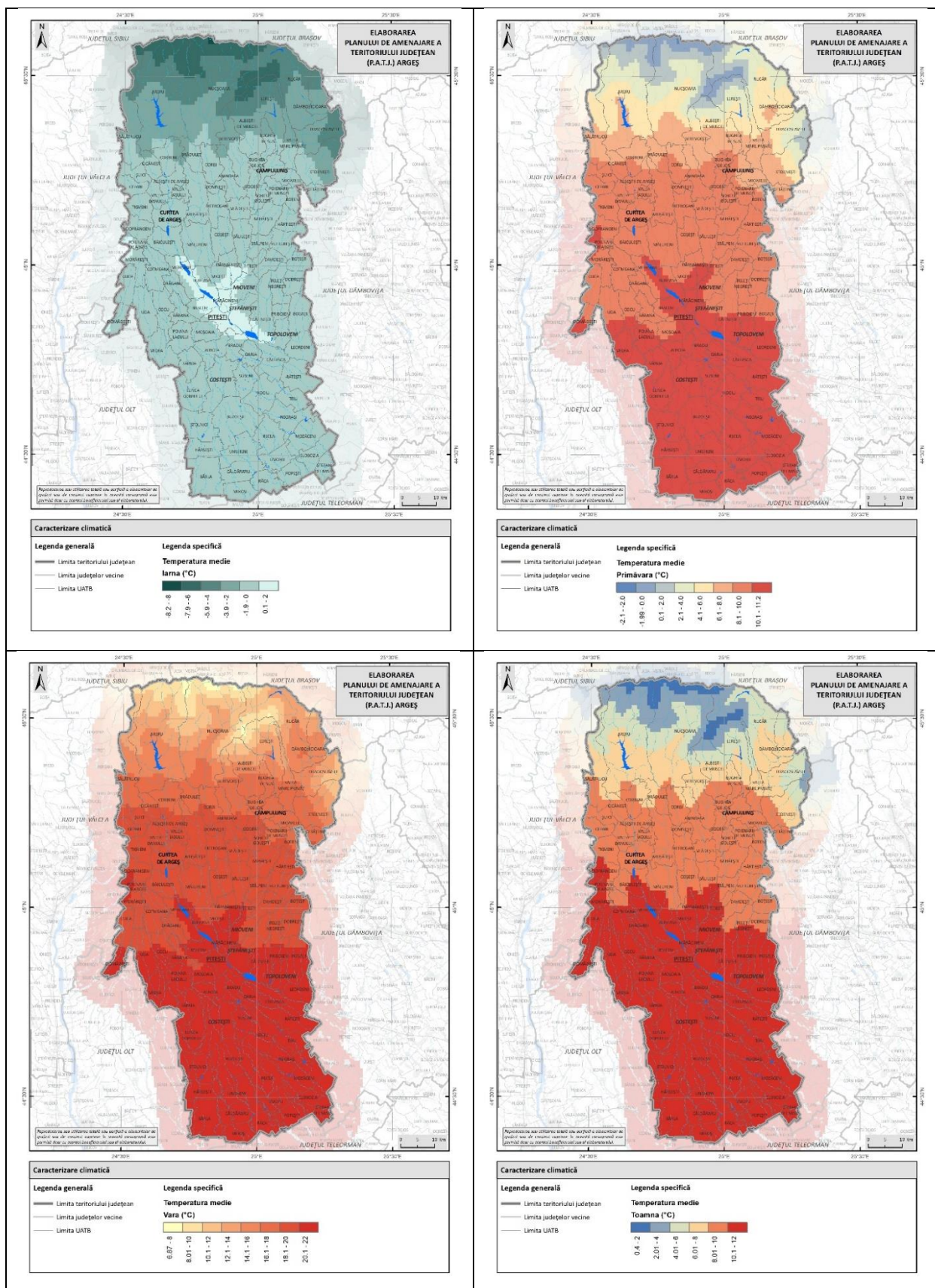
Fig. 2.7. TEMPERATURA MEDIE ANOTIMPUALĂ A AERULUI ÎN JUDEȚUL ARGEȘ PENTRU PERIOADA 1961-2023.
