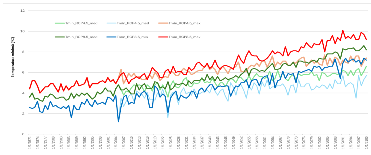
Fig. 2.20. EVOLUȚIA TEMPERATURII MINIME MODELATE ÎN SCENARIU RCP4,5 ȘI 8,5 ÎN JUDEȚUL ARGEȘ PENTRU PERIOADA 1971-2100.
