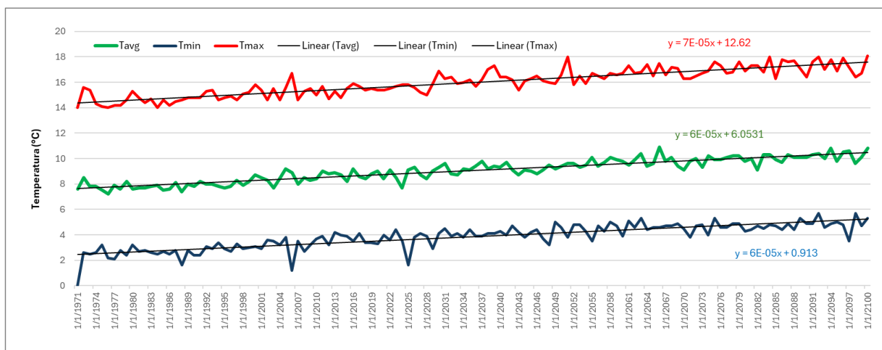
Fig. 2.9 EVOLUȚIA ASCENDENTĂ A TEMPERATURILOR MEDII ȘI EXTREME LA NIVELUL JUDEȚULUI ARGEȘ 1971-2100 SCENARIU RCP 4,5 ANM - www.roadapt.ro
