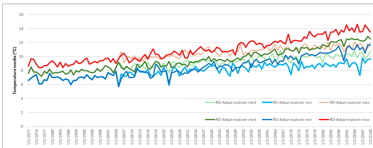
Fig. 2.21. EVOLUȚIA TEMPERATURII MEDII MODELATE ÎN SCENARIU RCP4,5 ȘI 8,5 ÎN JUDEȚUL ARGEȘ PENTRU PERIOADA 1971-2100.
