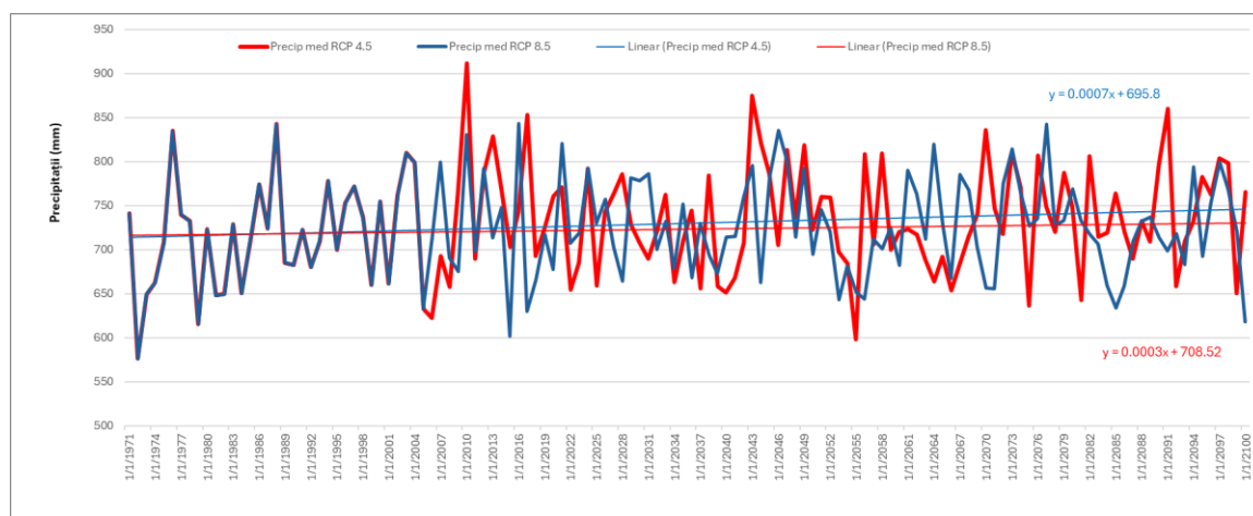
Fig. 2.22. EVOLUȚIA PRECIPITAȚIILOR MEDII MODELATE ÎN SCENARIU RCP4,5 ȘI RCP8,5 ÎN JUDEȚUL ARGEȘ PENTRU PERIOADA 1971-2100.
