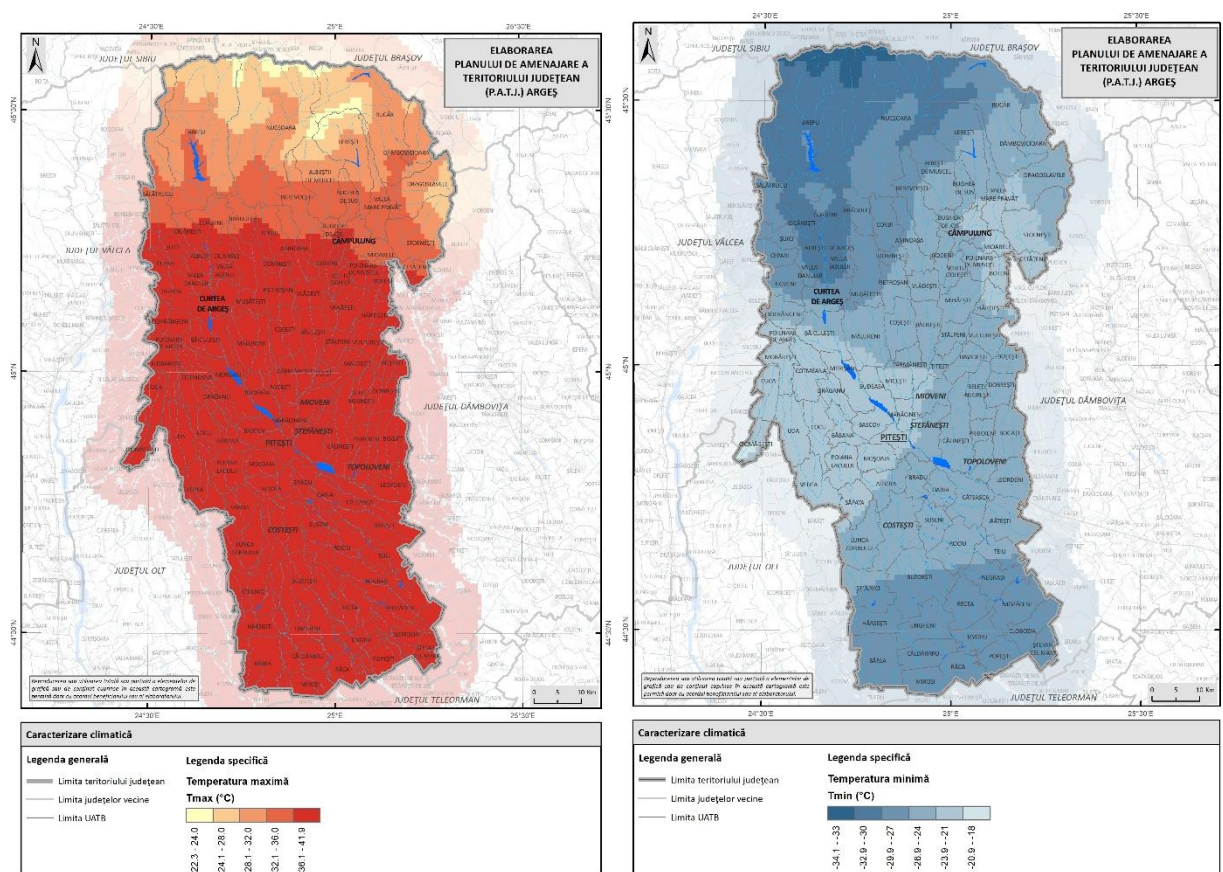
Fig. 2.8. TEMPERATURA MAXIMĂ (STÂNGA) ȘI MINIMĂ (DREAPTA) MULTIANUALĂ A AERULUI ÎN JUDEȚUL ARGEȘ 1961-2023.
