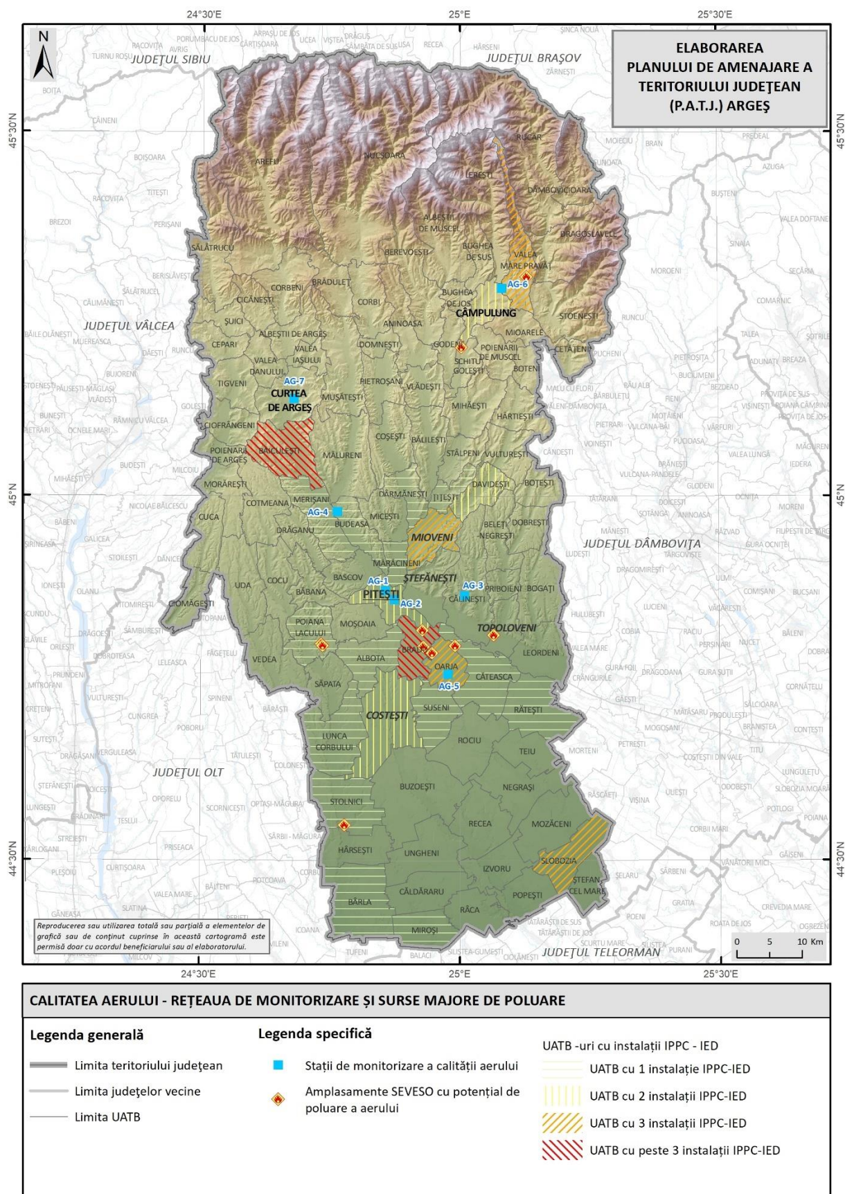
Fig. 2.40 CALITATEA AERULUI. SURSELE DE POLUARE ȘI REȚEAUA DE MONITORIZARE Sursa: Planul de menținere a calității aerului Argeș 2020-2024, Raportul anual starea mediului APM Argeș 2023, PAAR ISU Argeș
