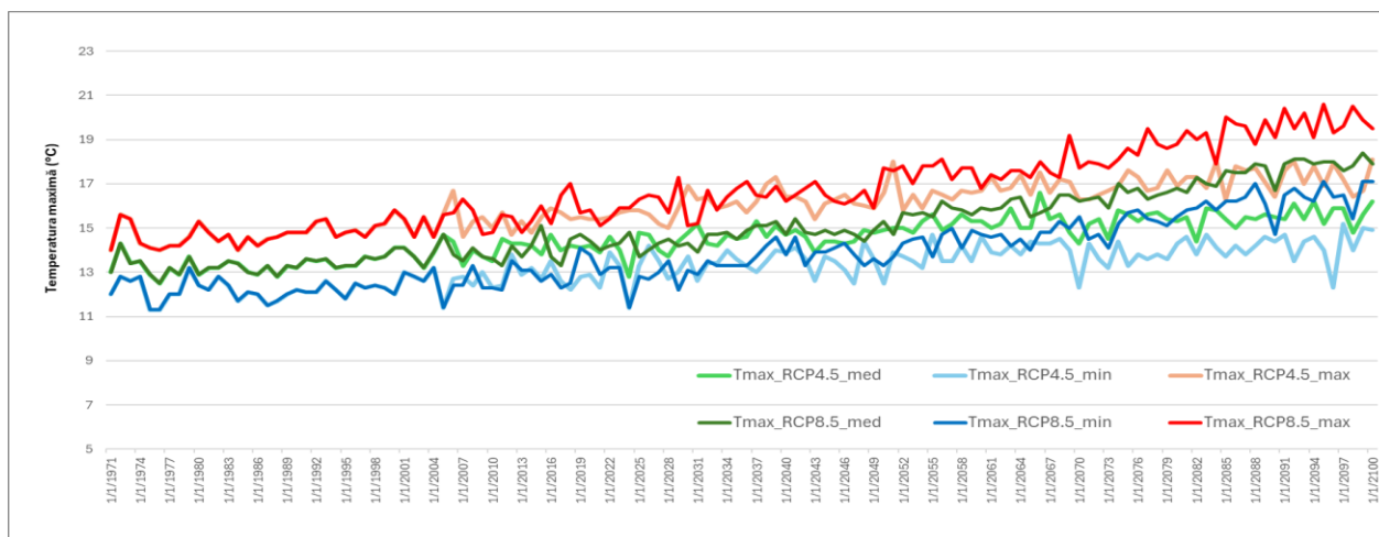
Fig. 2.19. EVOLUȚIA TEMPERATURII MAXIME MODELATE ÎN SCENARIU RCP4,5 ȘI 8,5 ÎN JUDEȚUL ARGEȘ PENTRU PERIOADA 1971-2100.
