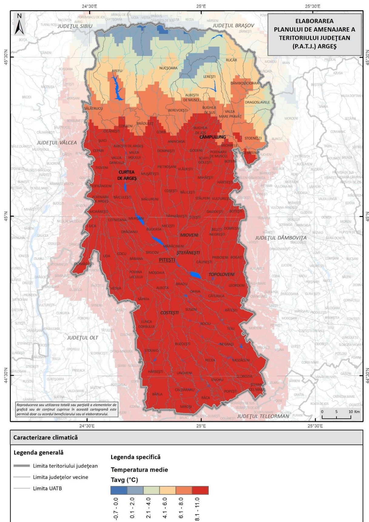
Fig. 2.6. TEMPERATURA MEDIE ANUALĂ A AERULUI ÎN JUDEȚUL ARGEȘ 1961-2023.
