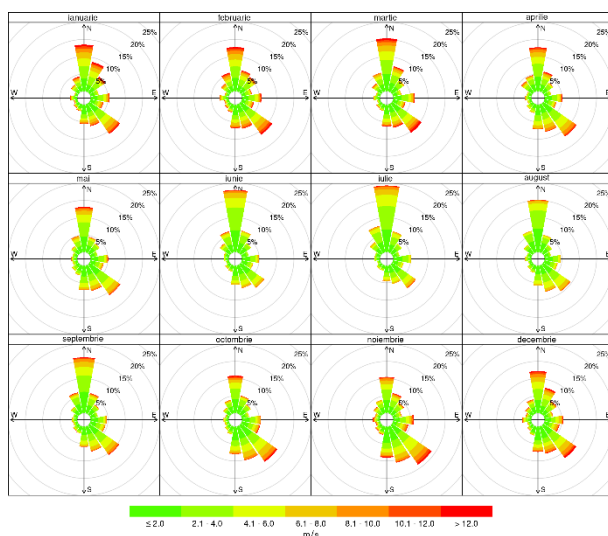
Stația meteorologică Bâlea Lac
