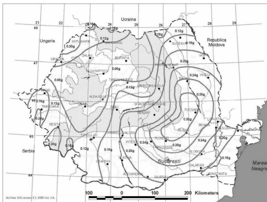
Fig. 2.44. ZONAREA TERITORIULUI ROMÂNIEI ÎN TERMENI DE VALORI DE VÂRF ALE ACCELAȚIEI TERENULUI PENTRU PROIECTARE AG PENTRU CUTREMURE AVÂND INTERVALUL MEDIU DE RECURENȚĂ IMR = 100 ANI
