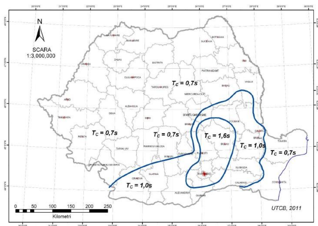
Fig. 2.43. HARTA ZONĂRII TERITORIULUI ÎN TERMENI DE PERIOADĂ DE COLȚ, T_C A SPECTRULUI DE RĂSPUNS (MDRAP, 2013).
