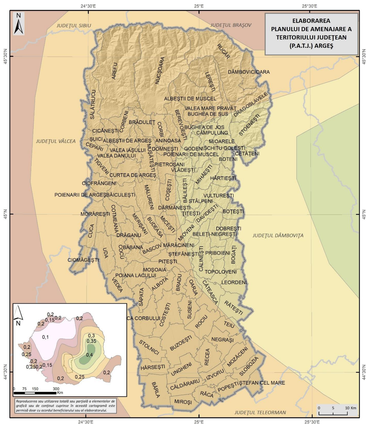
Harta zonării valorilor de vârf ale accelerației terenului pentru proiectare ag cu IMR = 225
