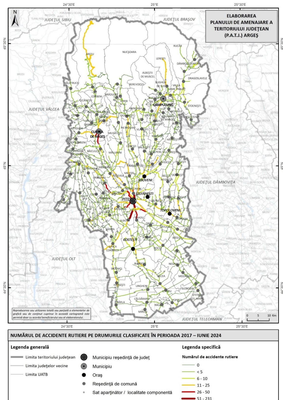
Fig. 2.30 DISTRIBUȚIA ÎN PLAN TERITORIAL A NUMĂRULUI DE ACCIDENTE RUTIERE PE DRUMURILE CLASIFICATE DIN JUDEȚUL ARGEȘ ÎN PERIOADA 2017 – IUNIE 2024
