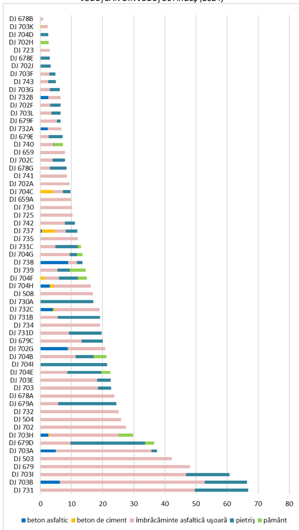
Fig. 2.14 STRUCTURA ÎMBRĂCĂMINȚII RUTIERE ȘI LUNGIMEA ACESTEIA PENTRU FIECARE DRUM JUDEȚEAN DIN JUDEȚUL ARGEȘ (2024)
