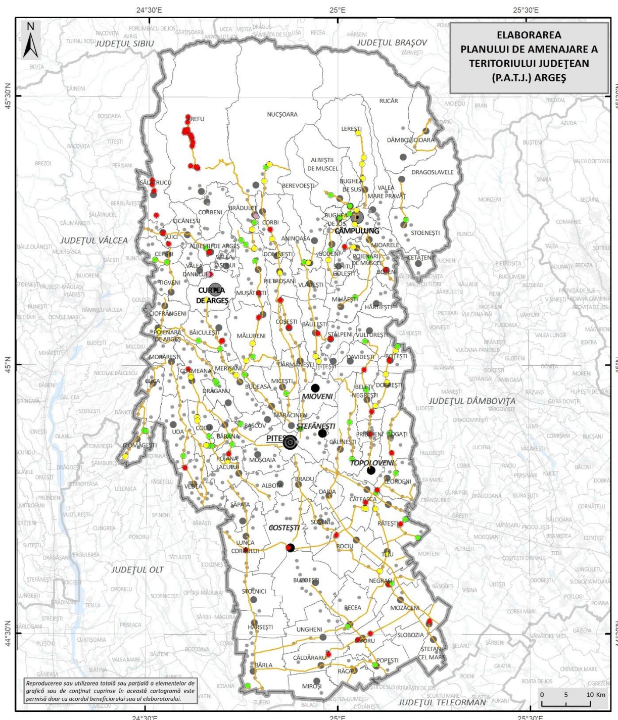
Fig. 2.21 DISTRIBUȚIA ÎN PLAN TERITORIAL A PODURILOR ȘI PODEȚELOR DE LA NIVELUL DRUMURILOR JUDEȚENE DIN JUDEȚUL ARGEȘ, DUPĂ STAREA DE VIABILITATE (2023)
