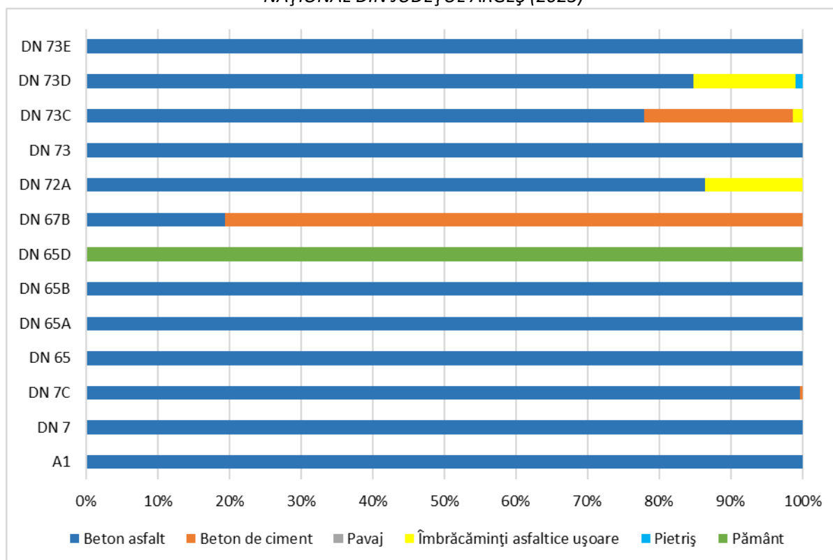
Fig. 2.12 STRUCTURA ÎMBRĂCĂMINȚII RUTIERE ȘI PONDEREA ACESTEIA DIN LUNGIMEA FIECĂRUI DRUM NAȚIONAL DIN JUDEȚUL ARGEȘ (2023)
