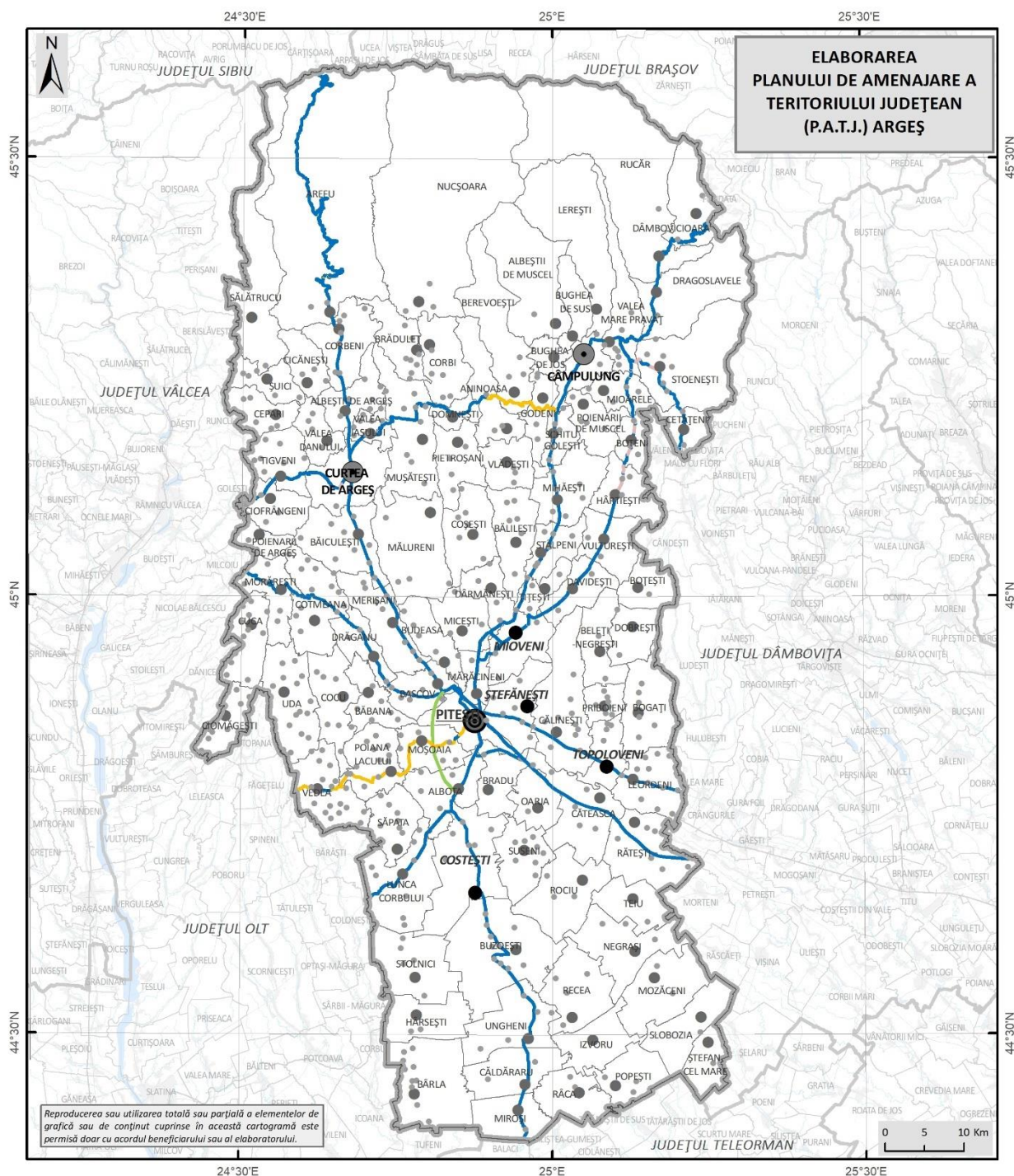
Fig. 2.13 DRUMURILE NAȚIONALE DIN JUDEȚUL ARGEȘ CLASIFICATE DUPĂ TIPUL ÎMBRĂCĂMINȚII ASFALTICE (2023)
