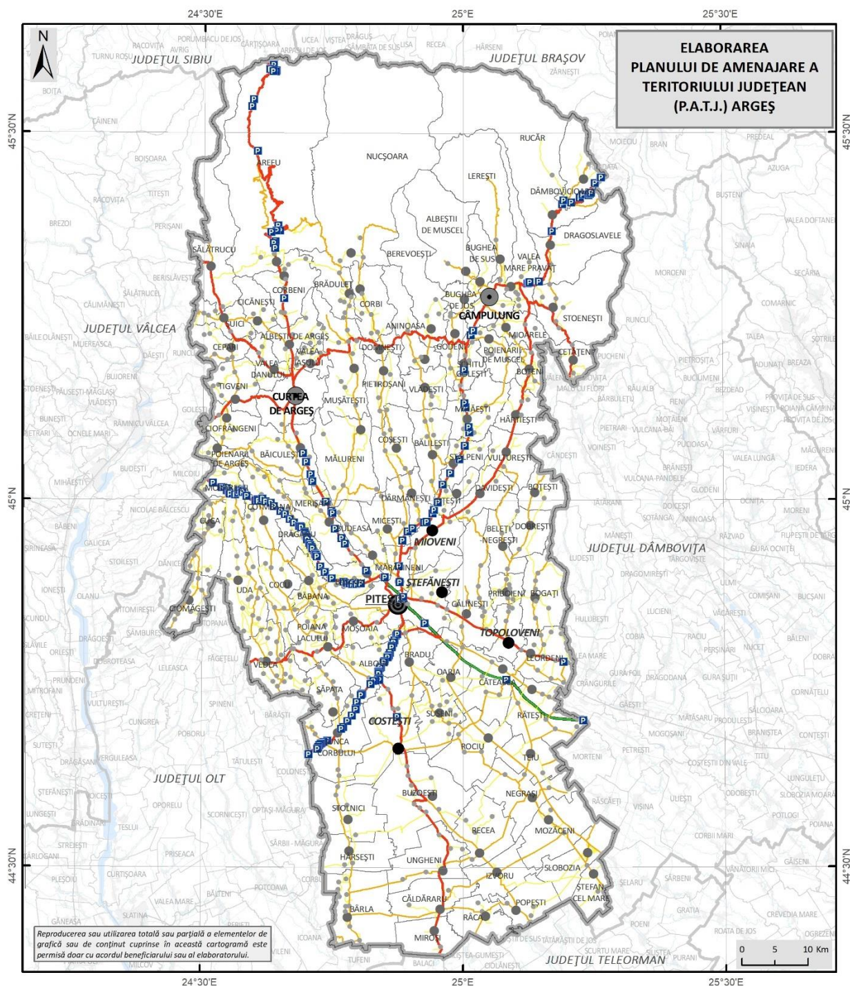
Fig. 2.26 DISTRIBUȚIA TERITORIALĂ A SPAȚIILOR DE PARCARE, OPRIRE ȘI STAȚIONARE DE PE REȚEAUA DE DRUMURI NAȚIONALE ȘI AUTOSTRĂZI DIN JUDEȚUL ARGEȘ (NOIEMBRIE 2024)
