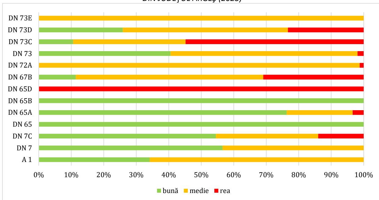
Fig. 2.17 STAREA DE VIABILITATE ȘI PONDERA ACESTEIA DIN LUNGIMEA FIECĂRUI DRUM NAȚIONAL DIN JUDEȚUL ARGEȘ (2023)
