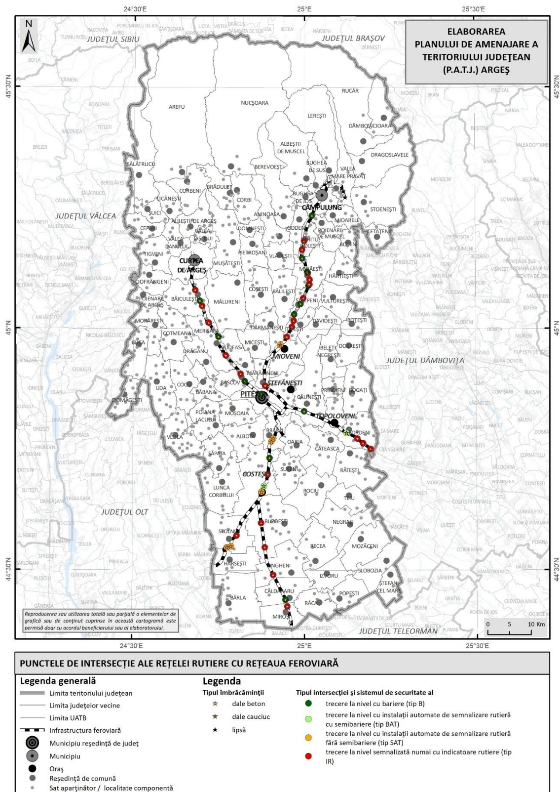
Fig. 2.23 PUNCTELE DE INTERSECȚIE ALE REȚELEI RUTIERE CU REȚEAUA FERROVIARĂ DIN JUDEȚUL ARGEȘ
