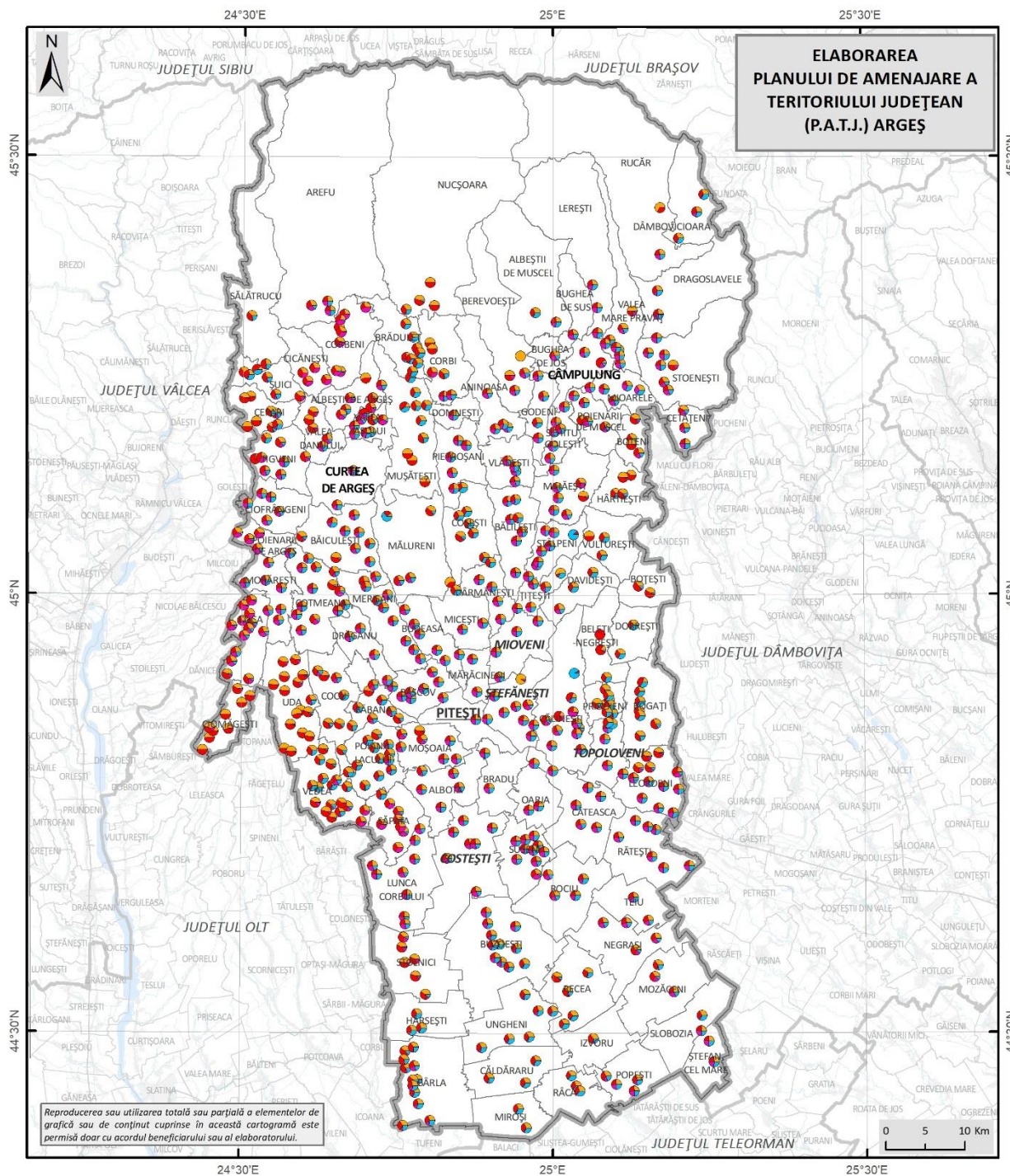
Fig. 2.48 ACOPERIRE CU SEMNAL PENTRU TEHNOLOGIA 3G
