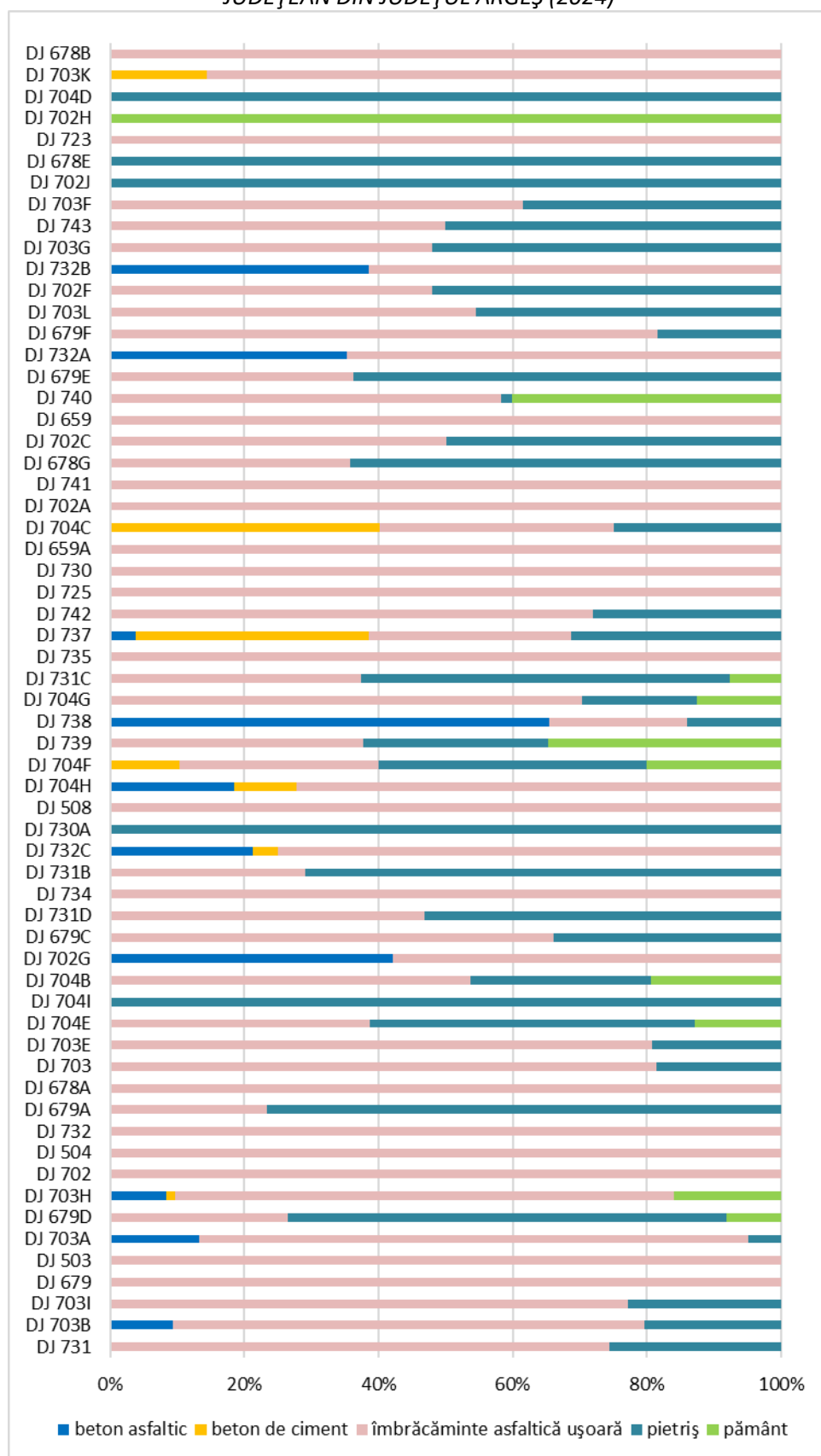
Fig. 2.15 STRUCTURA ÎMBRĂCĂMINȚII RUTIERE ȘI PONDEREA ACESTEIA DIN LUNGIMEA FIECĂRUI DRUM JUDEȚEAN DIN JUDEȚUL ARGEȘ (2024)
