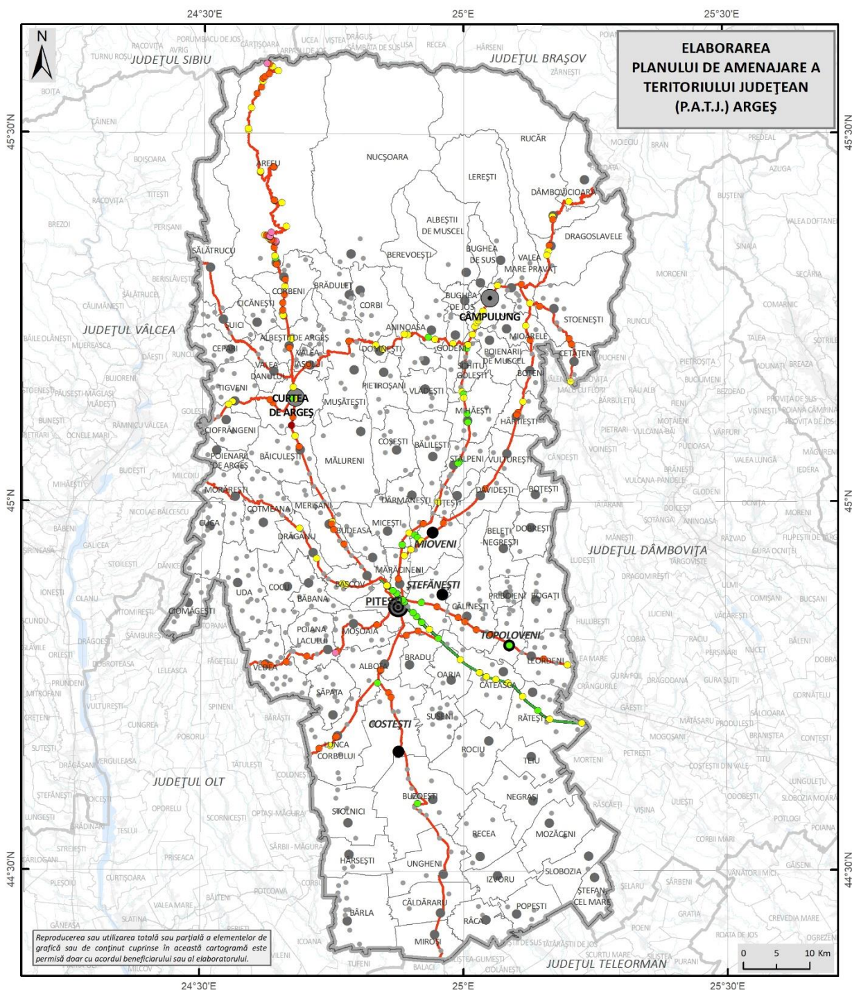
Fig. 2.19 DISTRIBUȚIA ÎN PLAN TERITORIAL A PODURILOR ȘI PODEȚELOR DE LA NIVELUL DRUMURILOR NAȚIONALE DIN JUDEȚUL ARGEȘ, DUPĂ STAREA DE VIABILITATE (2023)
