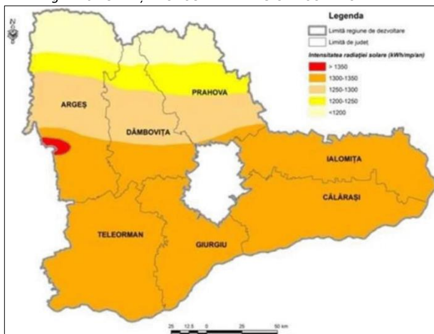
Fig. 2.46 POTENȚIALUL SOLAR AL REGIUNII SUD MUNTENIA
