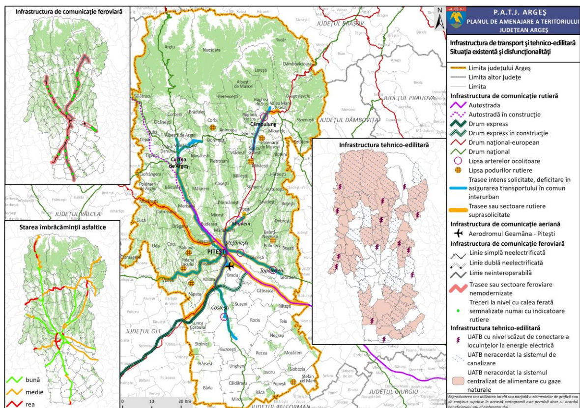
Fig. 3. INFRASTRUCTURA DE TRANSPORT ȘI TEHNICO-EDILITARĂ – SITUAȚIA EXISTENTĂ ȘI DISFUNȚIONALITĂȚI
